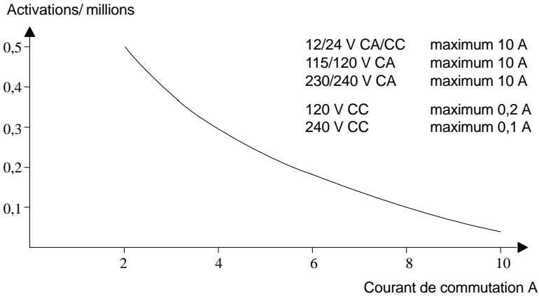
Figures A Caractéristiques de commutation et durée de vie des contacts en présence d'une charge ohmique (chauffe)
