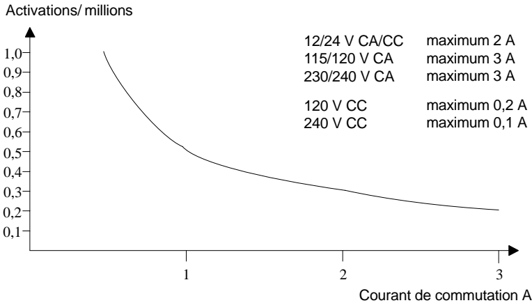
Figures B Caractéristiques de commutation et durée de vie des contacts en présence d'une forte charge inductive selon CEI 947-5-1 CC13/CA15 (contacteurs, bobines magnétiques, moteurs)
